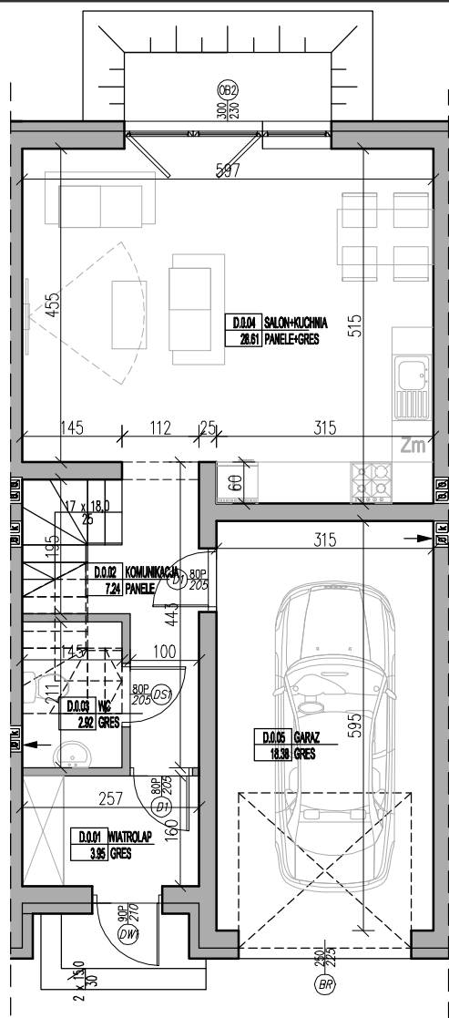
RZUT PARTERU LOKAL D
