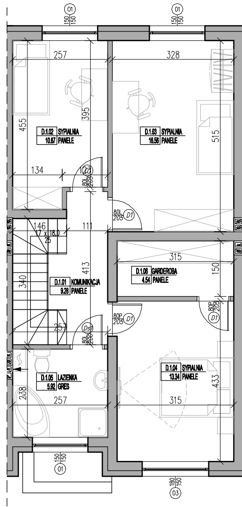
RZUT PIĘTRZA LOKAL D
