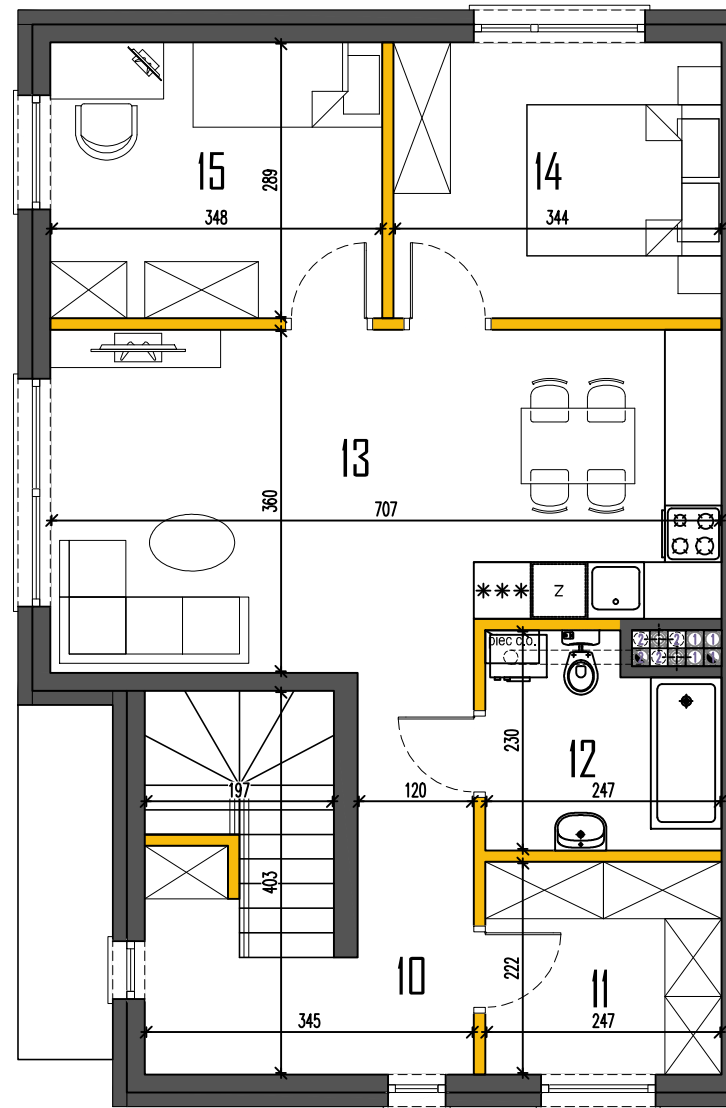
RZUT PIĘTRA
