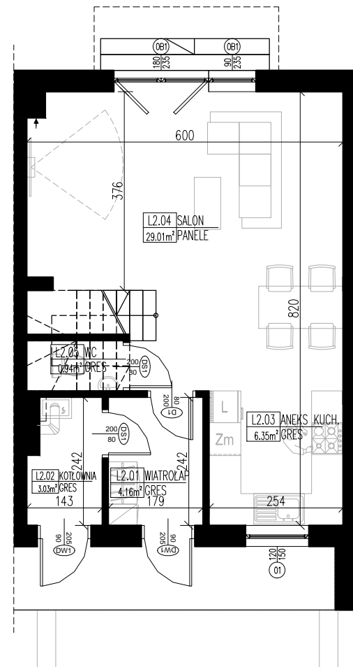
RZUT PARTERU
