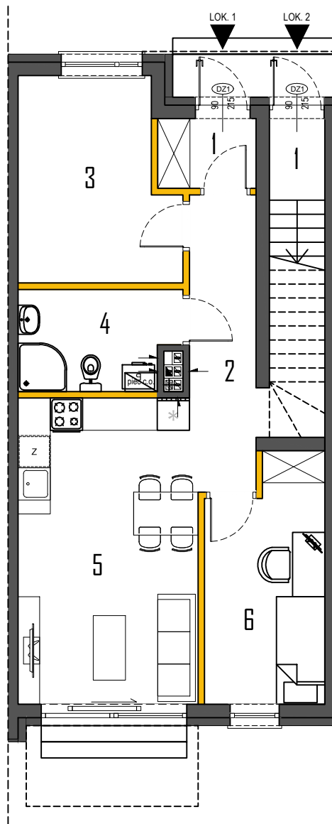
RZUT PARTERU
