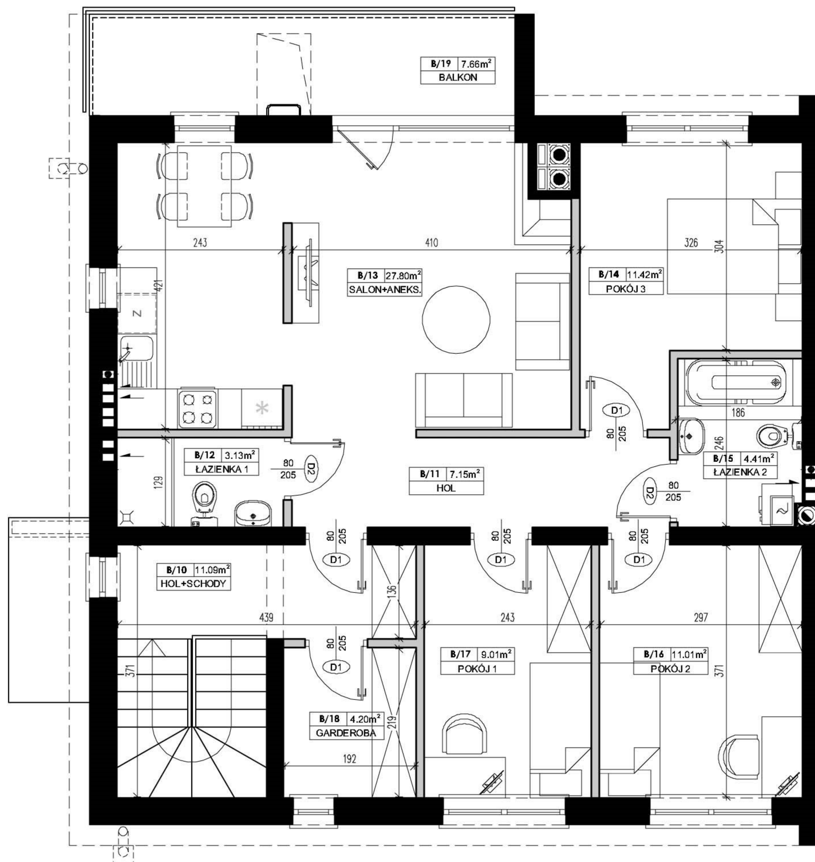
PIĘTRO
