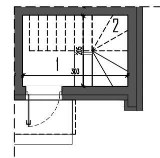
RZUT PARTERU
