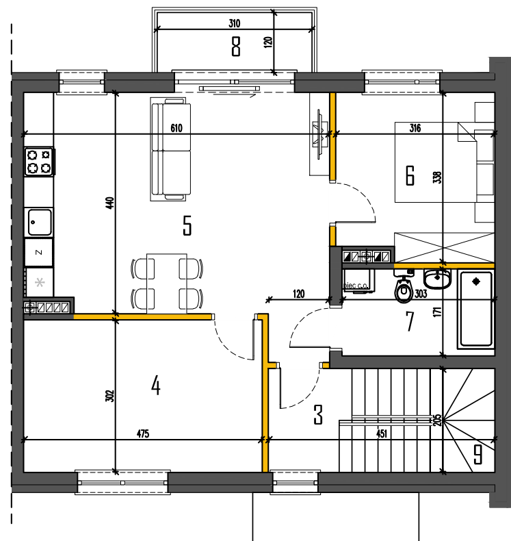
RZUT PIĘTRA
