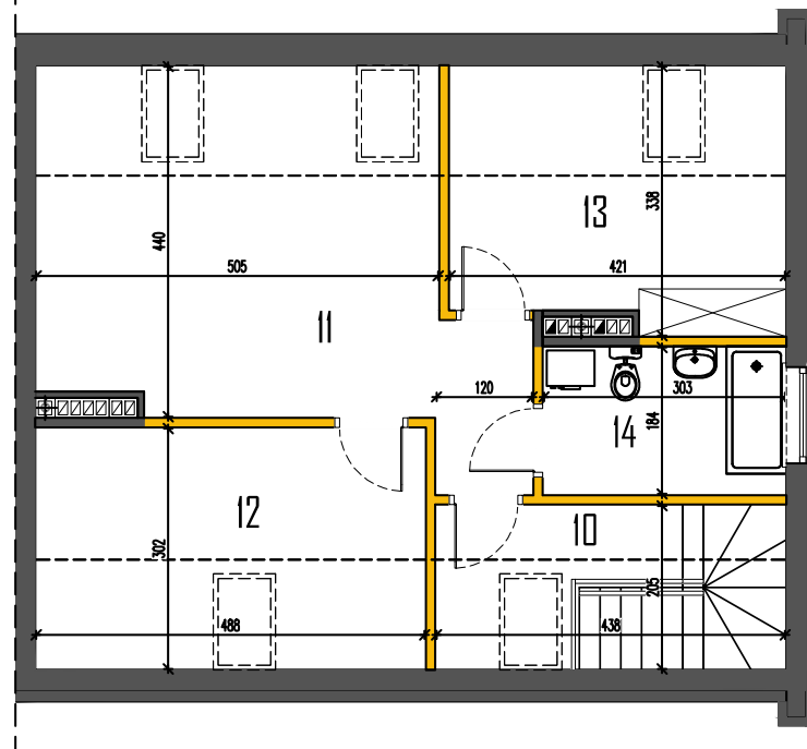
RZUT PODDASZA
