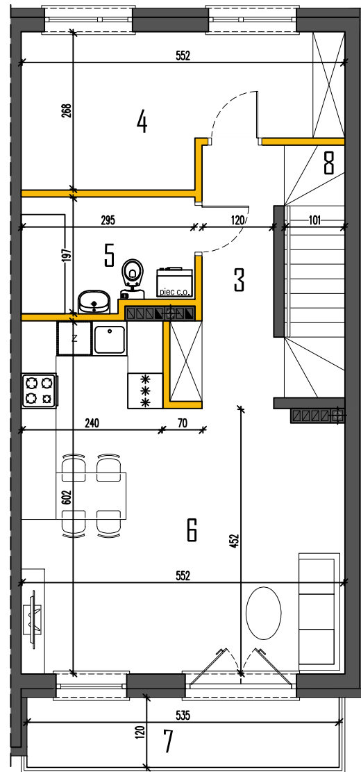
RZUT PIĘTRA
