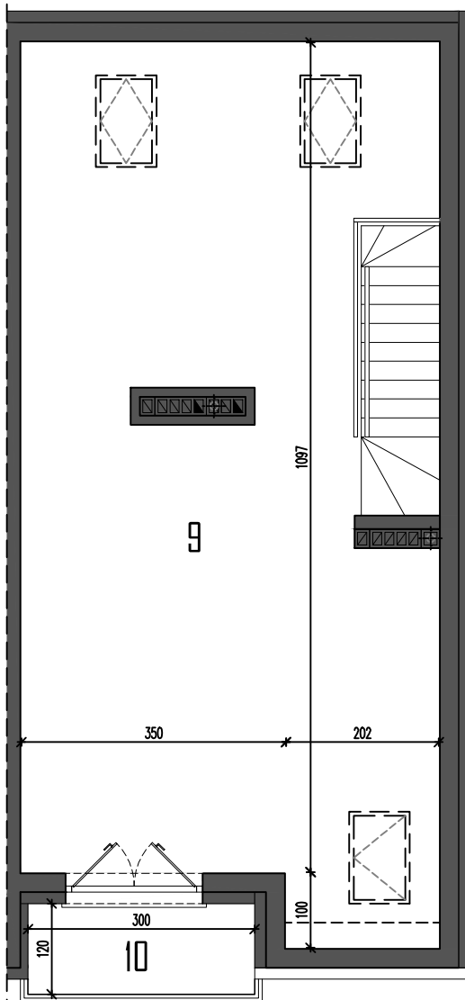
RZUT PODDASZA
