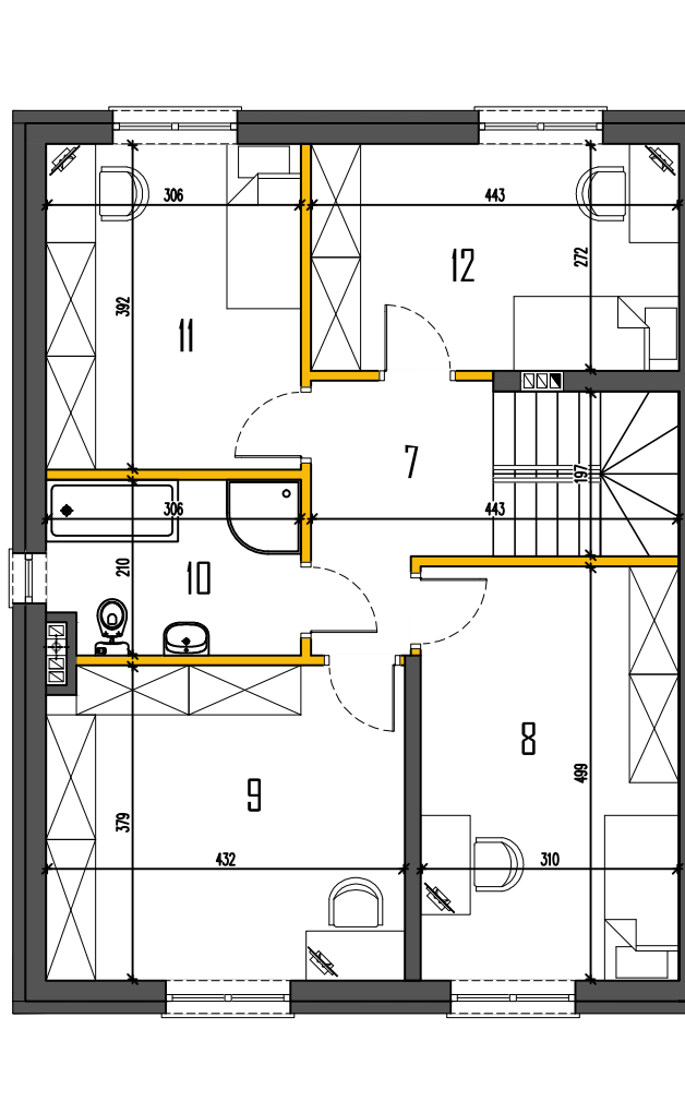
RZUT PIĘTRA
