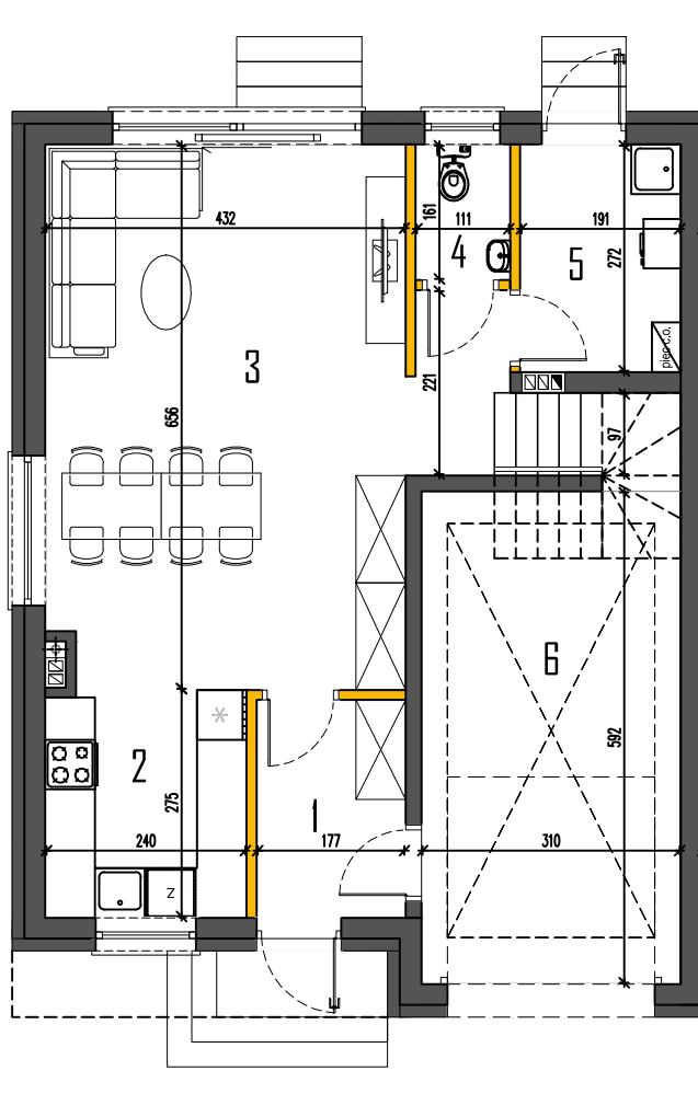
RZUT PARTERU
