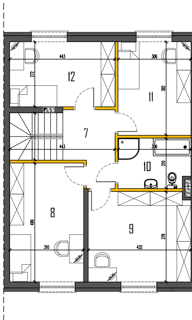
RZUT PIĘTRA
