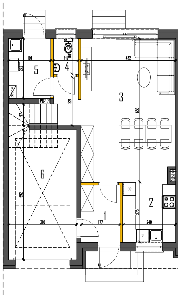
RZUT PARTERU
