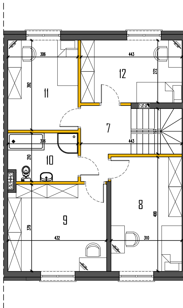
RZUT PIĘTRA
