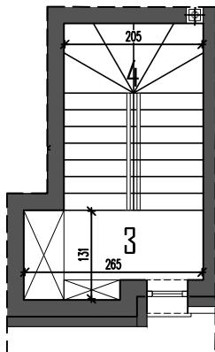
RZUT PIĘTRA
