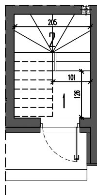
RZUT PARTERU
