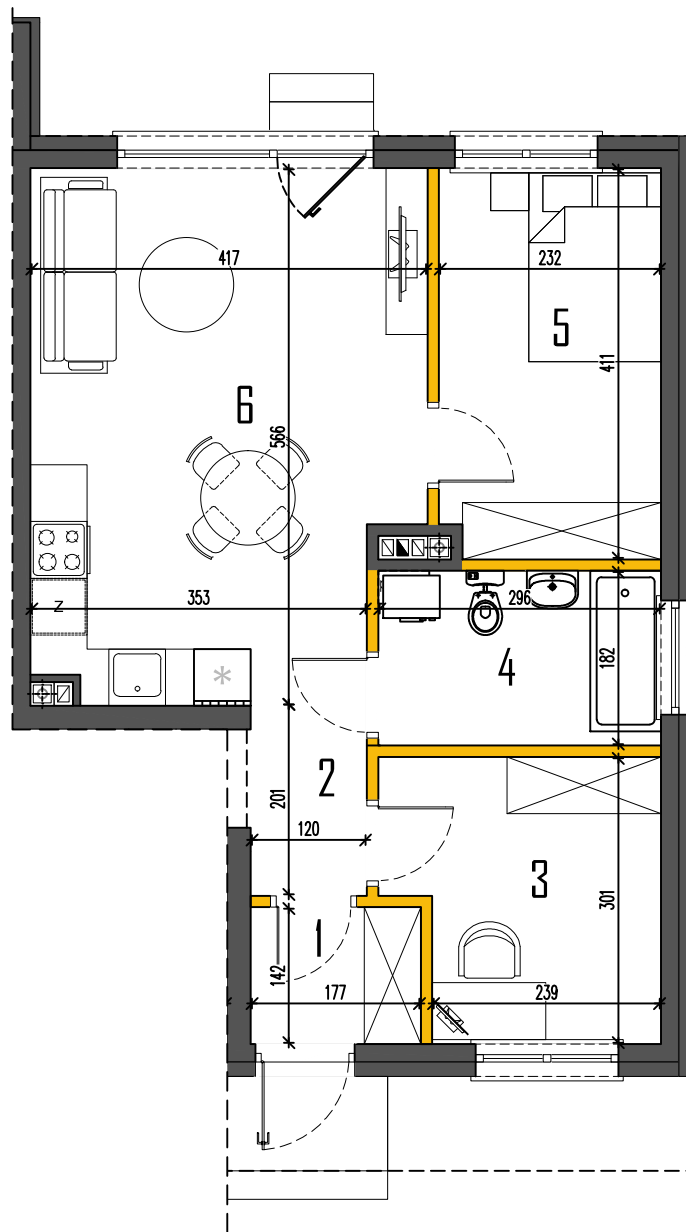
RZUT PARTERU
