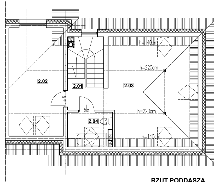
RZUT PODDASZA
