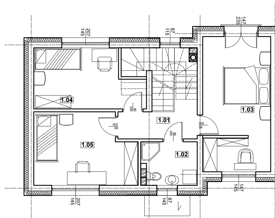
RZUT PIĘTRA
