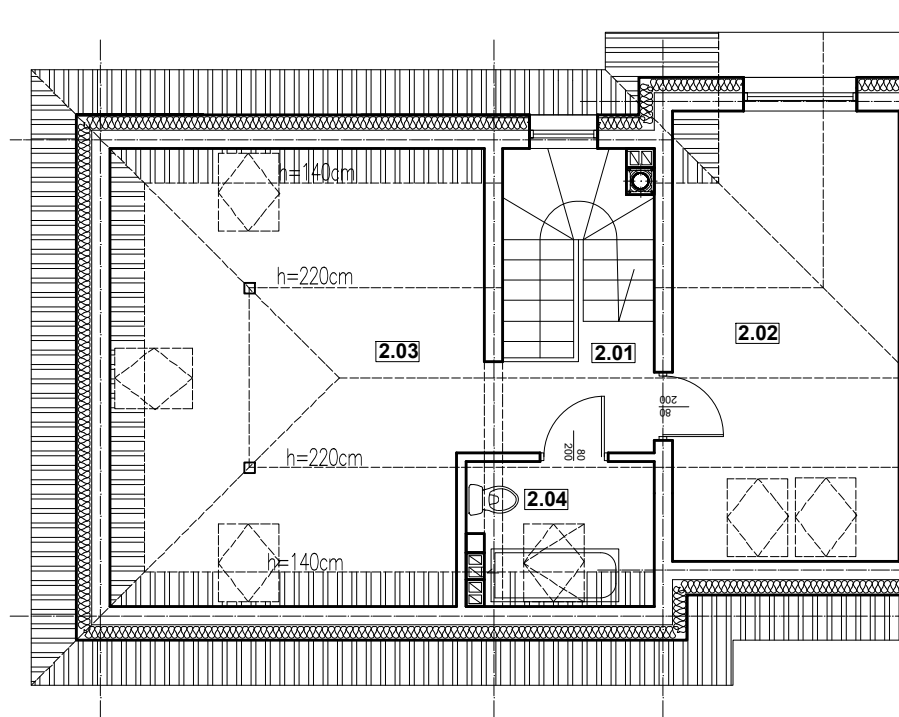
RZUT PODDASZA
