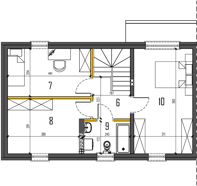
RZUT PARTERU
